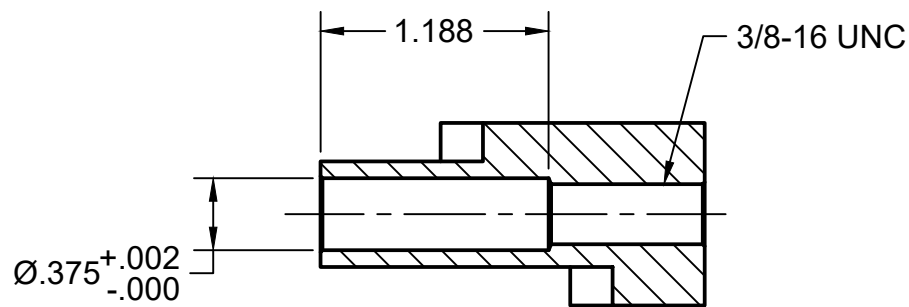
SECTION A-A SCALE 1:1
